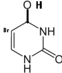
5-BU (énolique) : analogue de C
