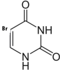
5-BU [cétonique] : analogue de T
